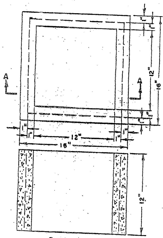
Section A-A BOX
