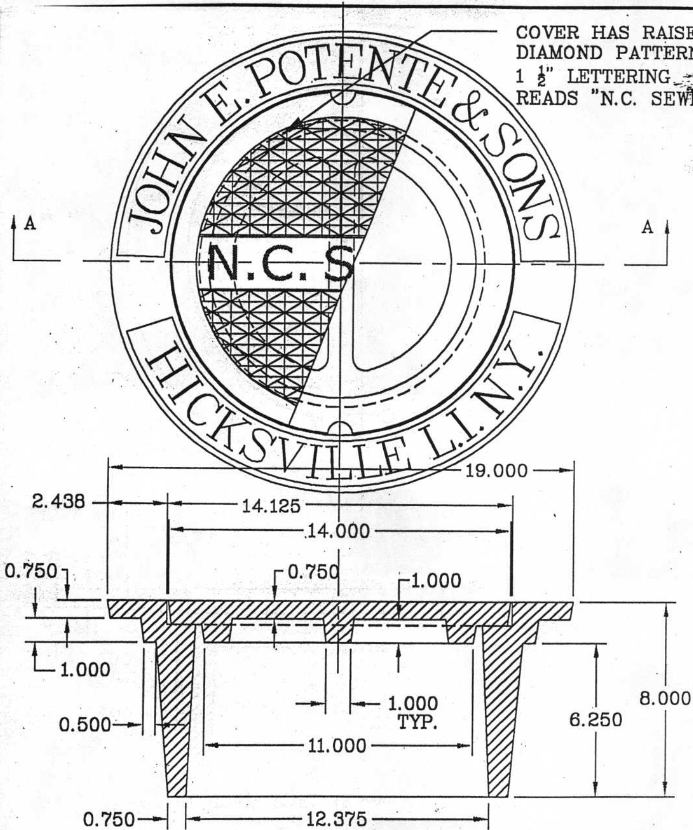
SECTION A-A
